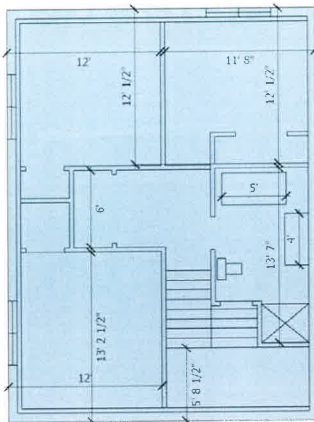
Plan sous-sol
